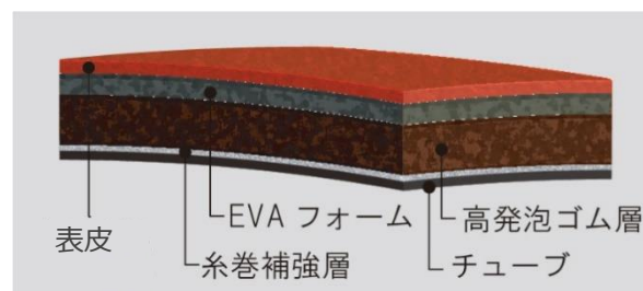
BG5000 の内部構造
